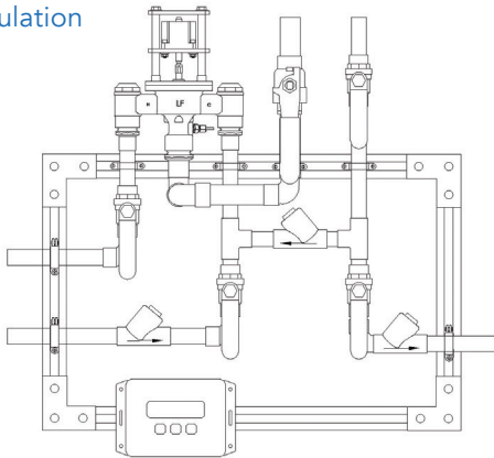
PNV-100-LF Proton Megatron
