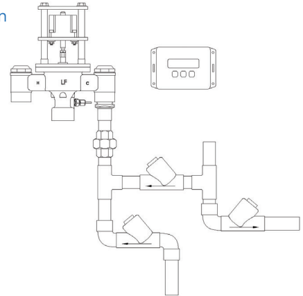
PNV-125-LF-R Simple Recirculation
